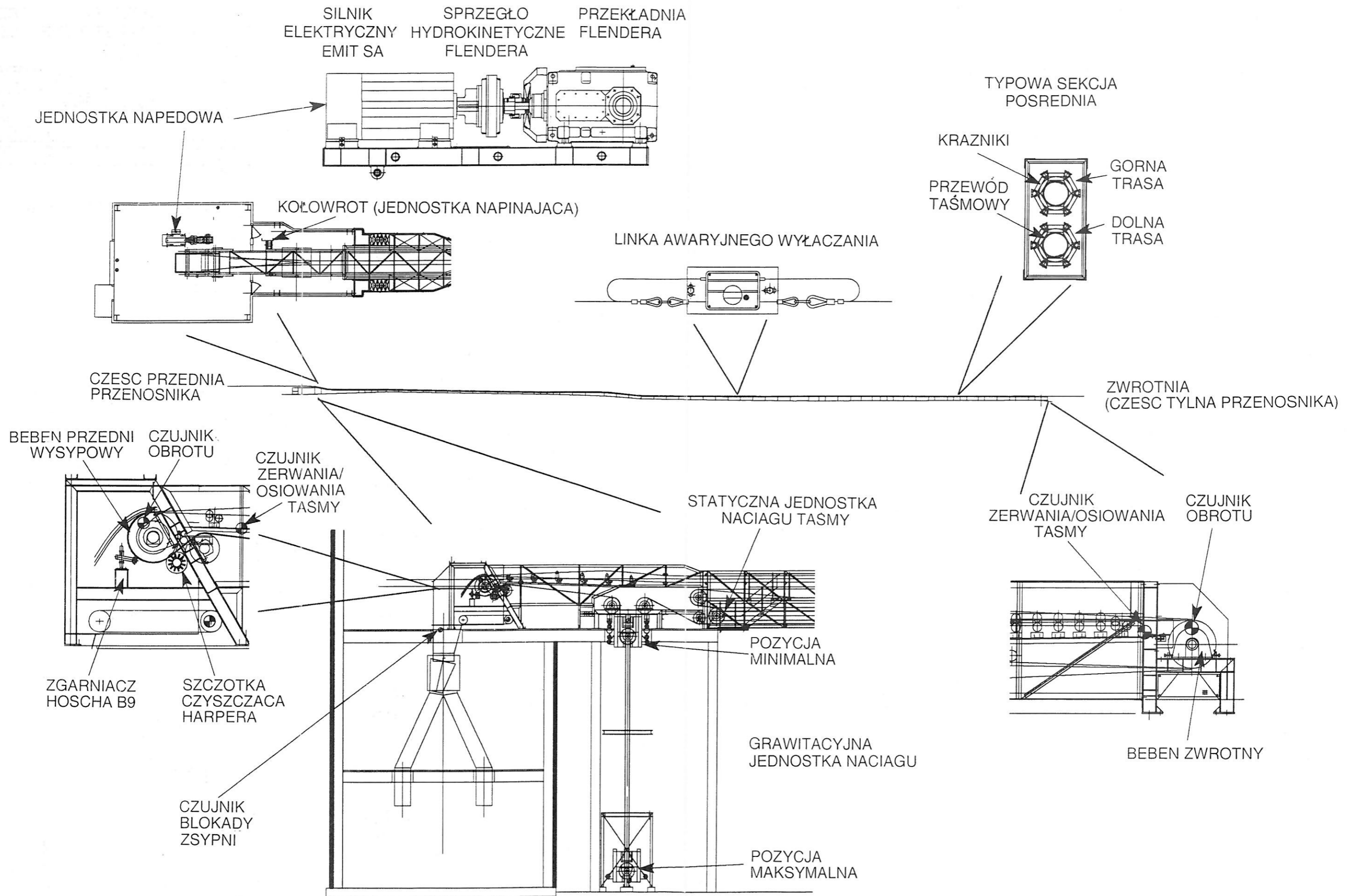
OGOLNY PLAN PRZENOSNIKA RUROWEGO
